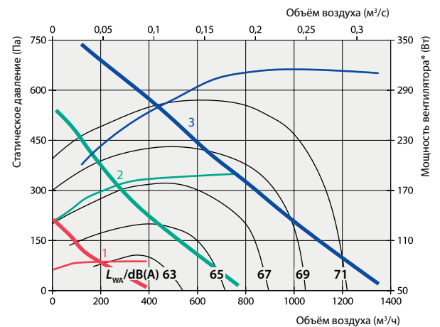
1, 2, 3 – скорость вентилятора*; – мощность вентилятора указана для одного вентилятора (потока). Данные производительности указаны для: вент. устройства с фильтром M5. Коэффициент коррекции для PW (водяного нагревателя) ~ 30 Па при 1200 м³/ч. Коэффициент коррекции для фильтра класса F7 ~ ~ 30 Па при 1200 м³/ч.
