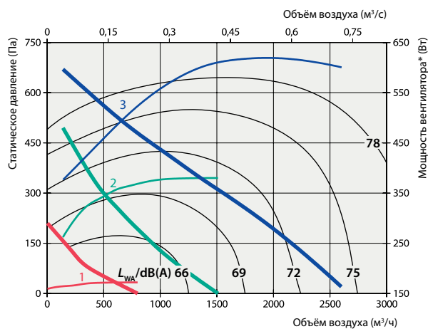
1, 2, 3 – скорость вентилятора*; – мощность вентилятора указана для одного вентилятора (потока). Данные производительности указаны для: вент. устройства с фильтром М5. Коэффициент коррекции для PW (водяного нагревателя) ~ 30 Па при 2000 м³/ч. Коэффициент коррекции для фильтра класса F7 ~ ~ 70 Па при 2000 м³/ч.
