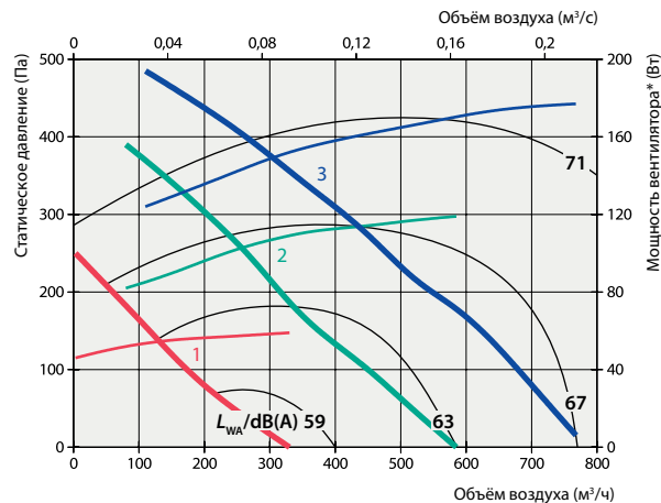
1, 2, 3 – скорость вентилятора*; – мощность вентилятора указана для одного вентилятора (потока). Данные производительности указаны для: вент. устройства с фильтром М5. Коэффициент коррекции для фильтра класса F7 – ~ 70 Па при 700 м 3 /ч.
