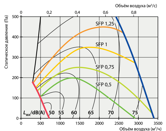
P[\text{кВт}] = \text{SFP}[\text{кВт}/(\text{м}^3/\text{с})] \cdot V[\text{м}^3/\text{с}] . На графике показан SFP одного вентилятора установки в которой фильтры класса M5. Коэффициент коррекции для фильтра класса F7 ~ ~ 70 Па при 3000 м³/ч.
