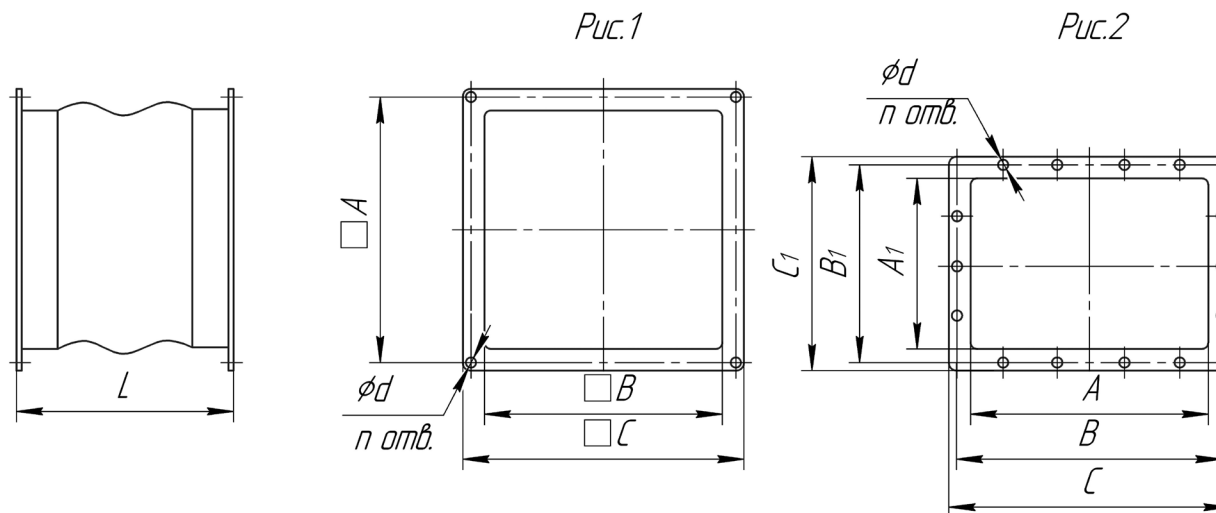
К вентиляторам ВР 85-77, ВР 280-46 (рис.1)
