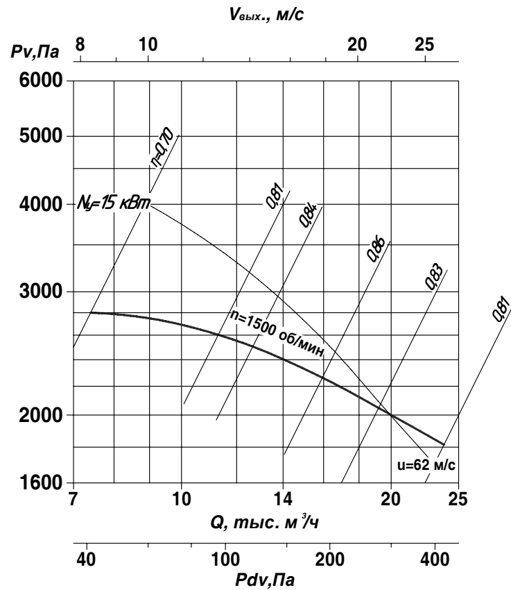
ВР 100-50(ВЦ5-50)-8 исп.1
