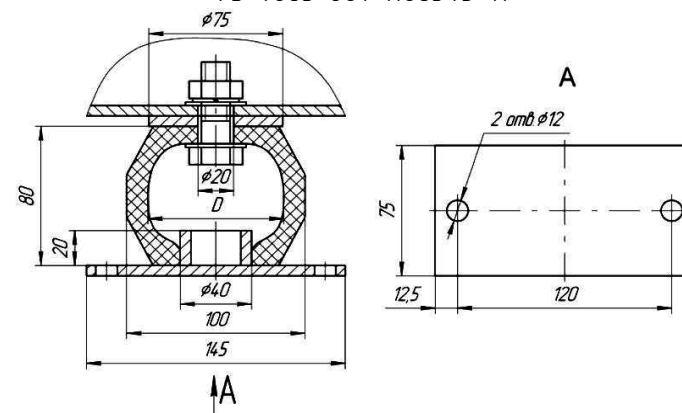
Виброизоляторы типа ВР
