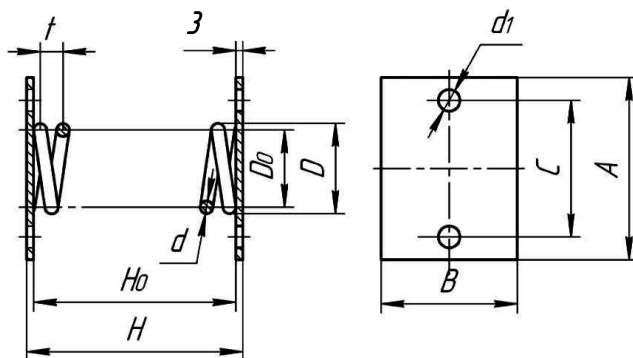
Виброизоляторы типа ДО, ВП
