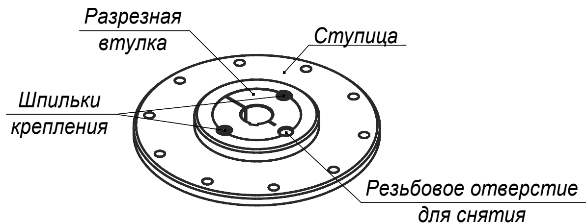
Рис. 27 – Быстросъемная ступица
