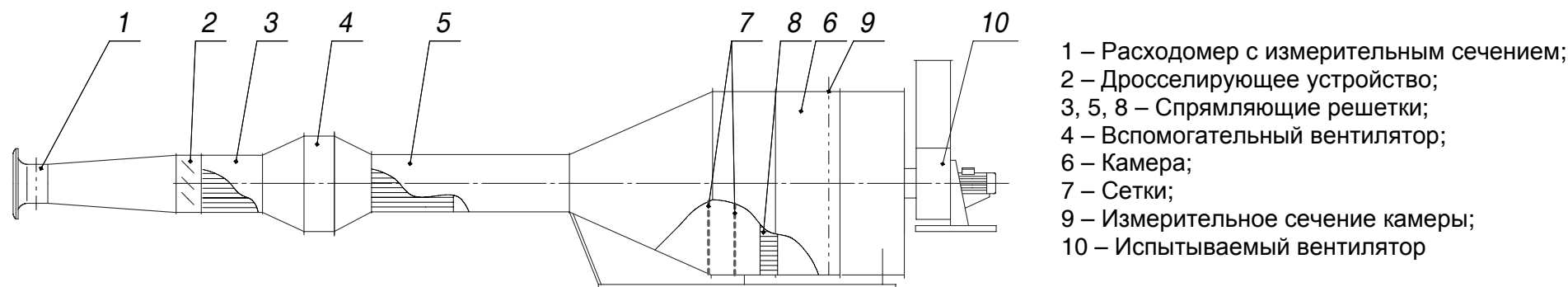
Рис. 3 – Схема стенда для аэродинамических испытаний
